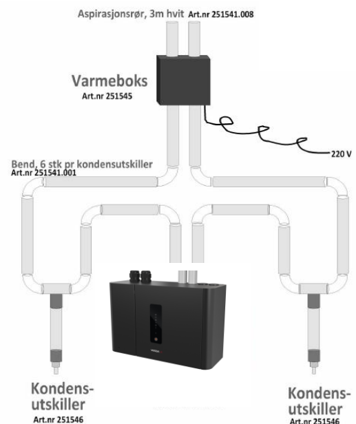
Eksempel på kobling av varmeboks og kondensutskiller
